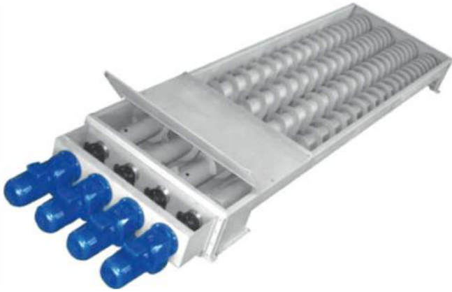
Treme Havuzu Kademeli Boşaltma Helezonu Treme Pondage Stepping Discharge Screw Conveyor حلزون نقل متعدد مخصص لنقل الأوحال
