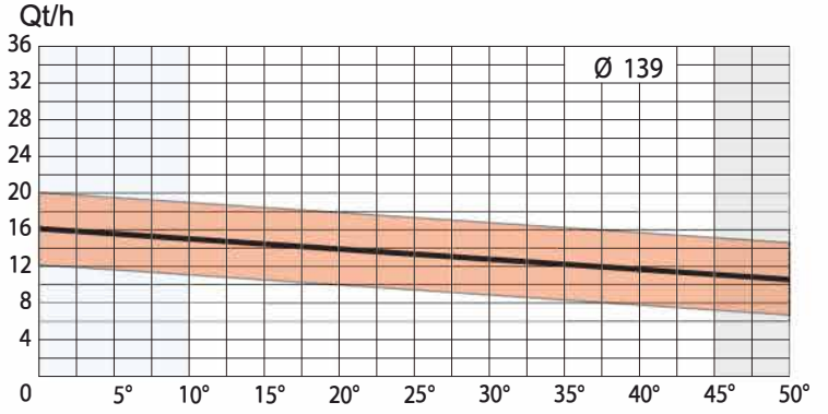
Çimento Helezonları Kapasite Tablosu Cement Screw Conveyor Capacity Table جدول الإستطاعة (الإنتاجية)
