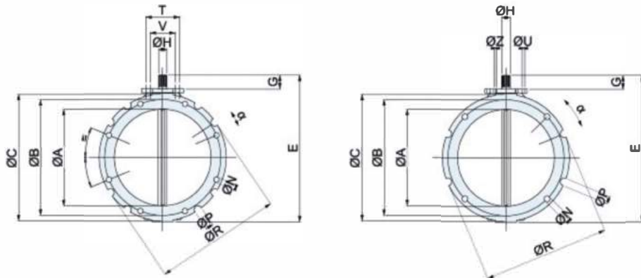
Tek Flanş / Single Flange / فلانجة مفردة
