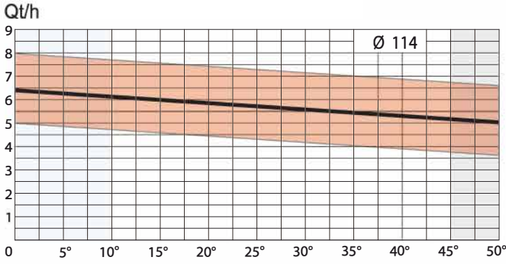
Çimento Helezonları Kapasite Tablosu Cement Screw Conveyor Capacity Table جدول الإستطاعة (الإنتاجية)
